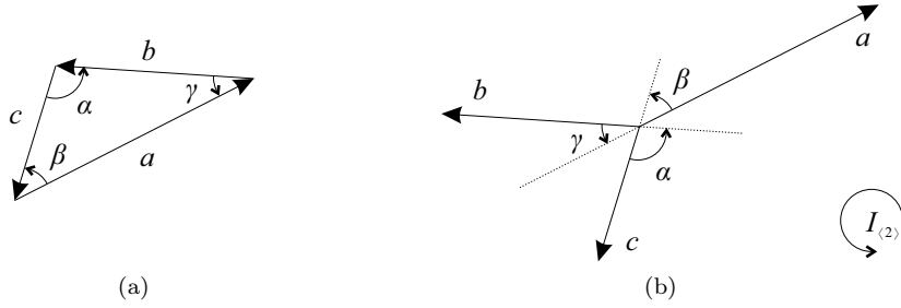
Figura 4.1: Um triângulo a + b + c = 0 no plano orientado I_{(2)} pode ser desenhado em sua forma clássica (a) ou na forma de vetores em um espaço vetorial (b).
