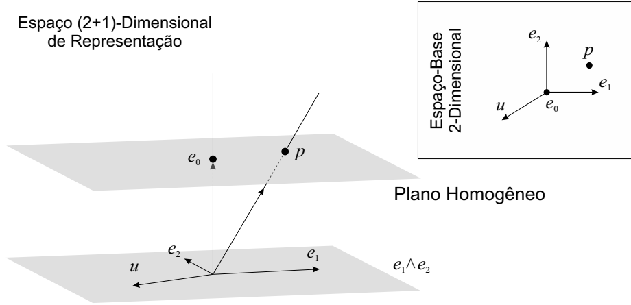
Figura 3.2: O plano paralelo a e_1 \wedge e_2 é a representação homogênea do espaço-base 2-dimensional, exibido como um espaço Cartesiano na imagem em detalhe, à direita. No modelo homogêneo, a interpretação geométrica de blades que residem no espaço (2 + 1)-dimensional de representação é dada pela intersecção dos blades com o plano homogêneo. Por exemplo, os vetores e_0 e p são interpretados como pontos próprios no espaço-base. Enquanto que os vetores e_1 , e_2 e u são interpretados como pontos impróprios, ou direções, por estarem contidos em e_1 \wedge e_2 .
