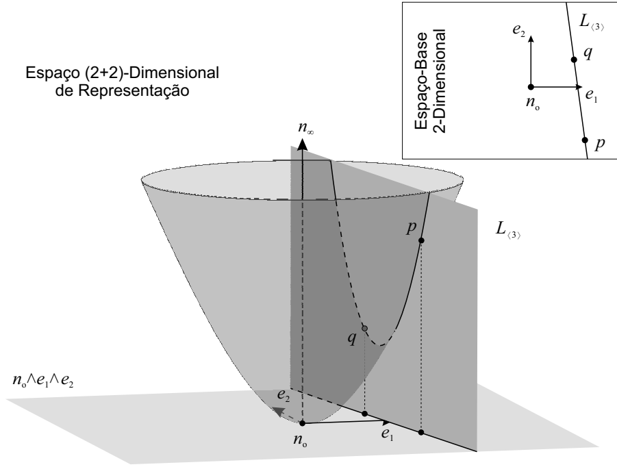
Figura 3.8: Quando um 3-blade define um plano paralelo a n_{\infty} na visualização homogênea do espaço de representação (e.g., L_{(3)} = p \wedge q \wedge n_{\infty} ), a interseção desse plano com o parabolóide de pontos finitos resulta em uma parábola. A projeção ortográfica dessa parábola no espaço-base faz com que o 3-blade seja geometricamente interpretado como uma reta.
